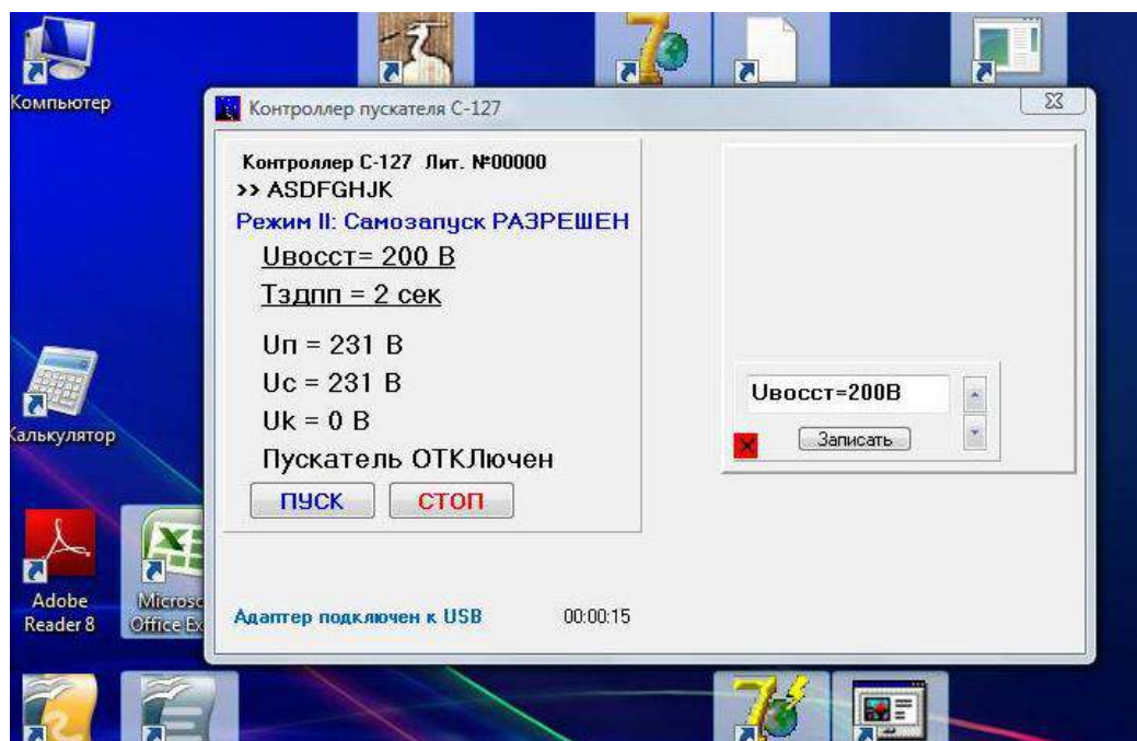
Рисунок 7 – окно корректировки настроек параметров контроллера СМАРТРЕЛЕ C-127
