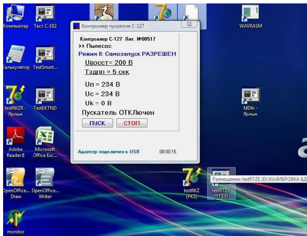
Рисунок 6 – окно отображения настроек параметров контроллера СМАРТРЕЛЕ C-127
